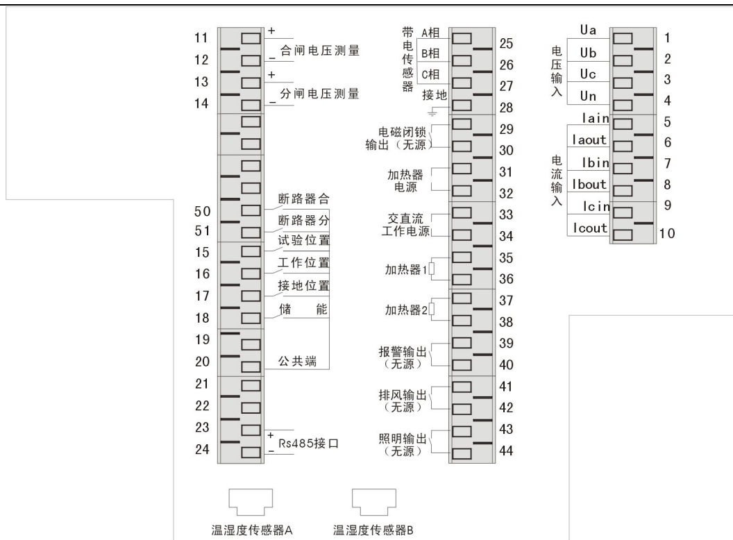
端子接线图
