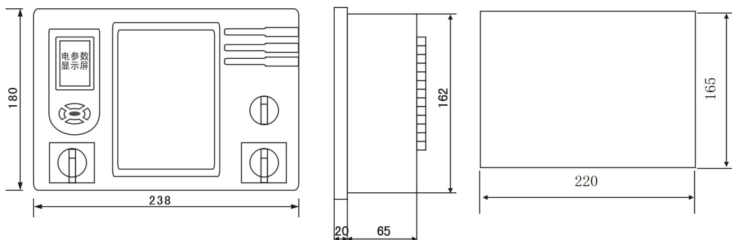
产品尺寸（正视）
