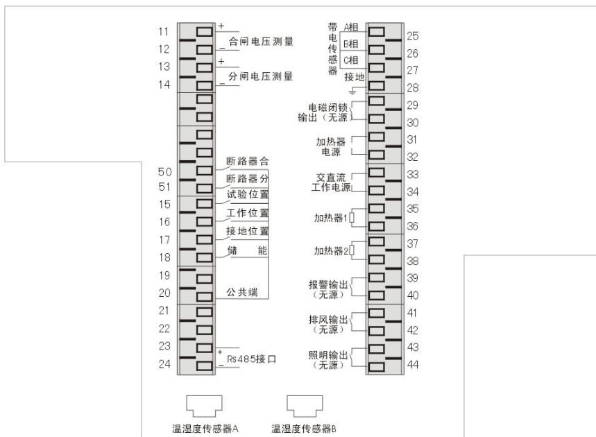
端子接线图
